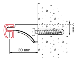
Wandmontage met wandsteun 2151.
