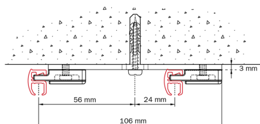
Voor goede parallele plaatsing: montage met dubbeldrager 2216 en plafondsteunen 2150.
