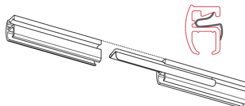
2152 railverbinder Toepassing van metalen verbinder in de rug van de 2102.
