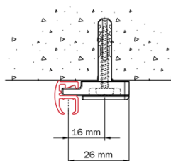
Plafondmontage met plafondsteun 2150.
