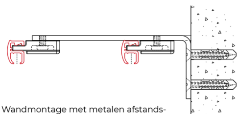
Wandmontage met metalen afstandsteunen en plafondsteunen 2150.
